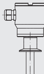
Клэмповое трубное соединение по DIN 32676
